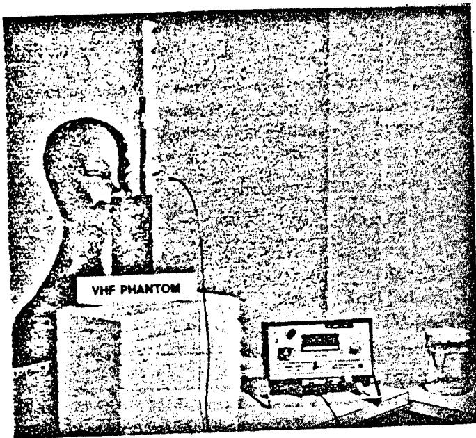
Fig. 2. Head phantom.
