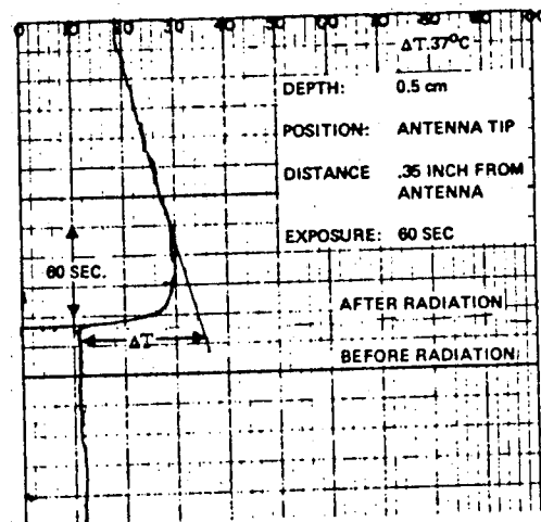
Fig. 3. Experimental data.
