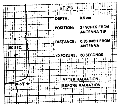
Fig. 3. Experimental data.
